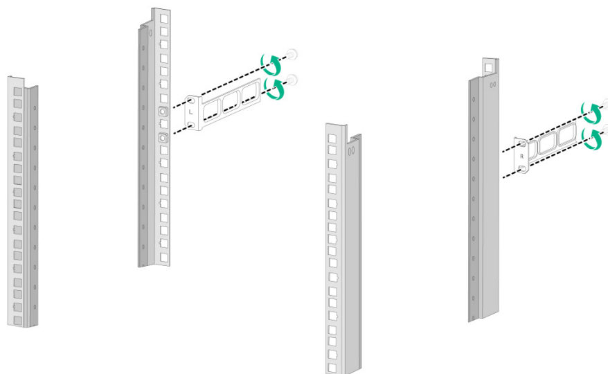
图2-4 安装后挂耳（后挂耳反装）
