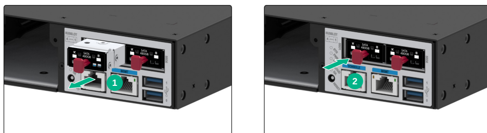
图2-12 安装硬盘
