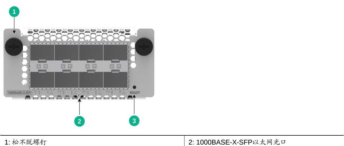
图1-4 NS-HPIM-GP8B-Z 接口模块正视图
