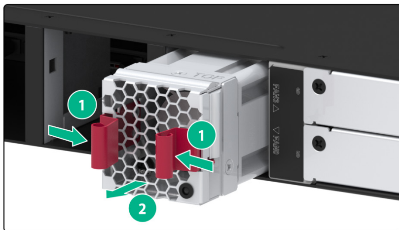
图4-1 风扇模块拆卸示意图
