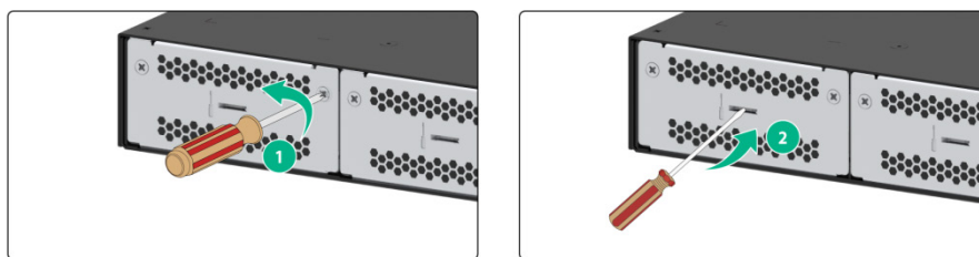
图2-10 拆卸假面板
