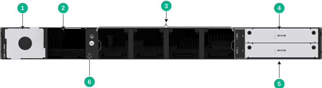
图1-2 设备后视图
