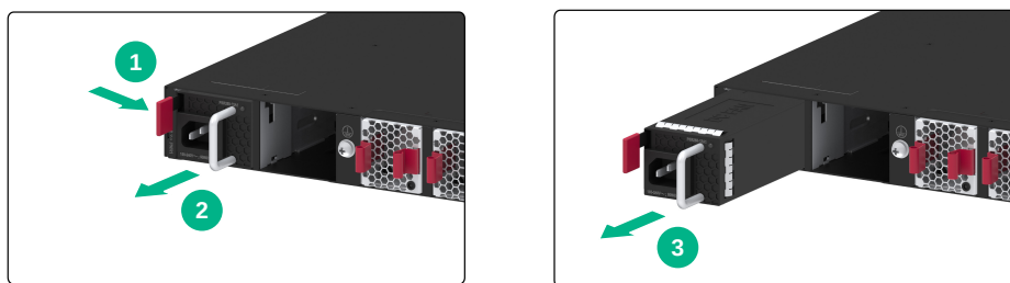
图4-2 拆卸电源模块
