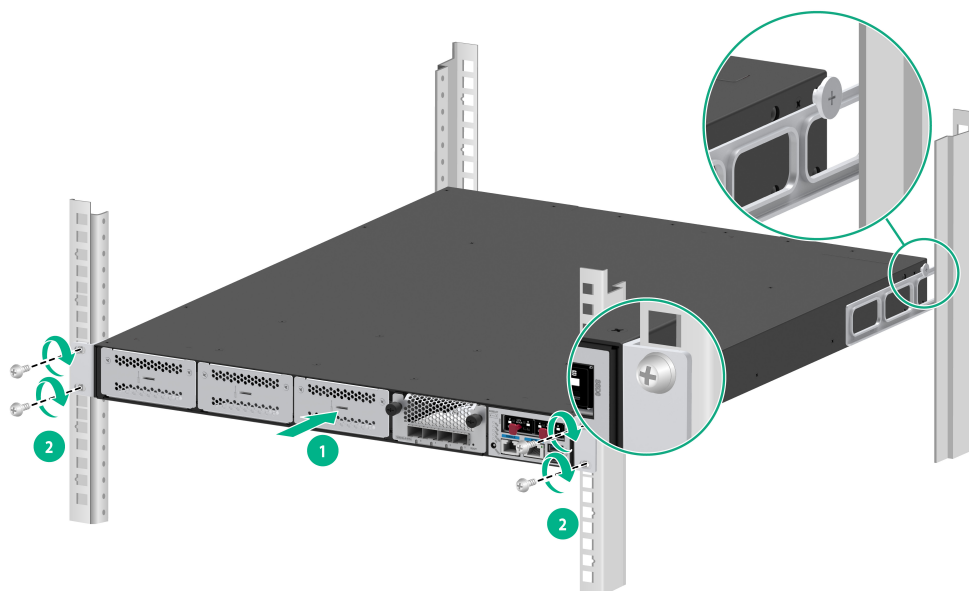
图2-5 安装设备到机柜（后挂耳正装）
