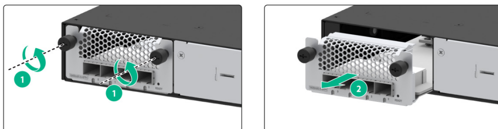
图4-3 拆卸接口模块
