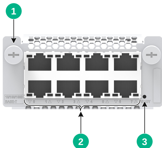
图1-5 NS-HPIM-GT8B-Z 接口模块正视图
