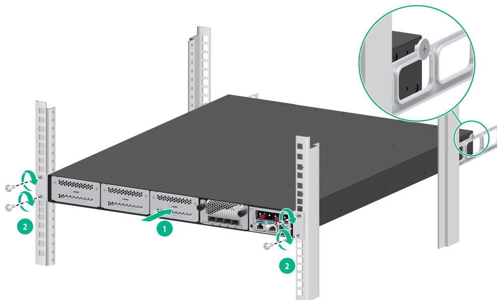
图2-6 安装设备到机柜（后挂耳反装）
