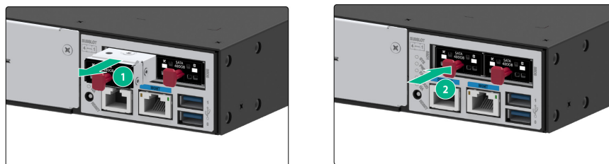
图4-4 更换硬盘
