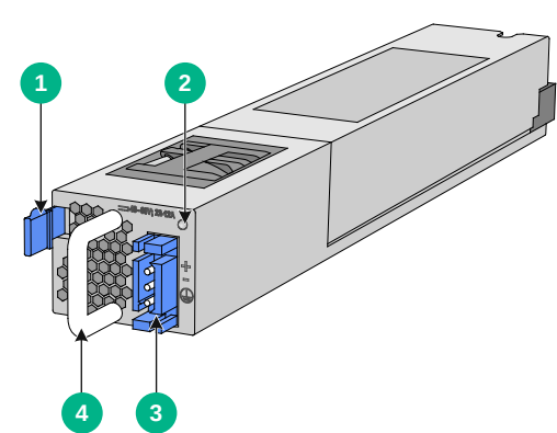
图1-7 直流电源模块正视图
