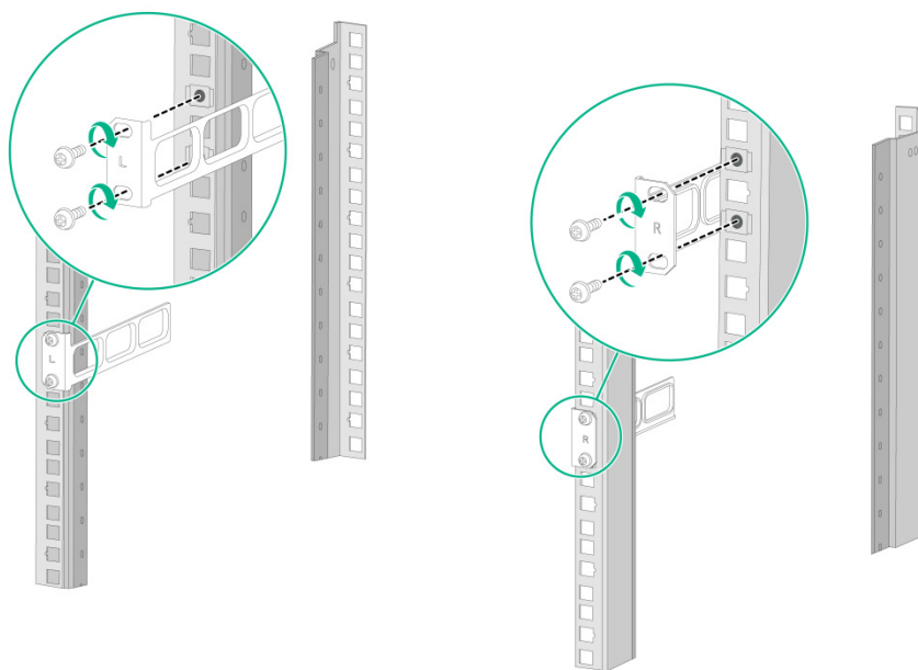
图2-3 安装后挂耳（后挂耳正装）
