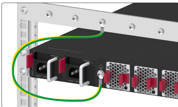
图2-7 连接到机柜接地
