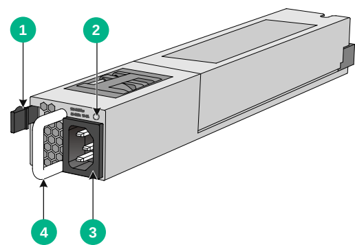
图1-6 交流电源模块正视图
