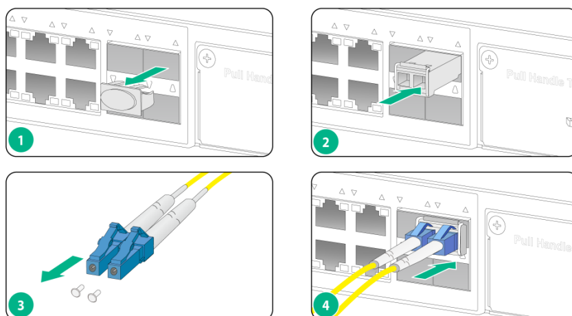
图2-15 安装及连接光模块
