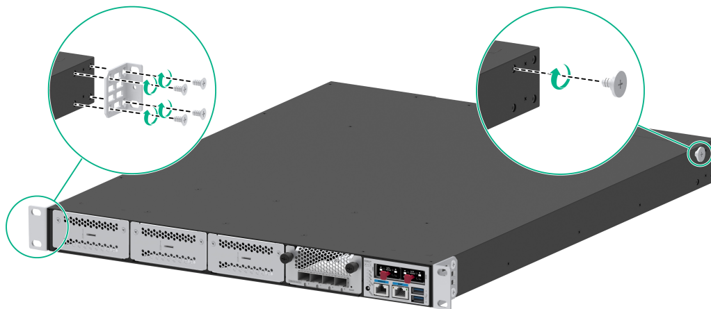
图2-2 安装前挂耳和承重螺钉
