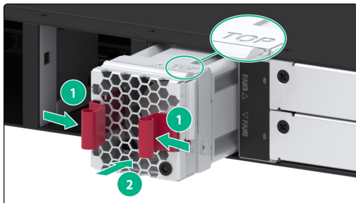
图2-8 风扇模块安装示意图
