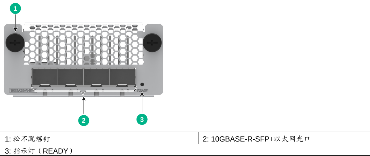
图1-3 NS-HPIM-TG4B-Z 接口模块正视图
