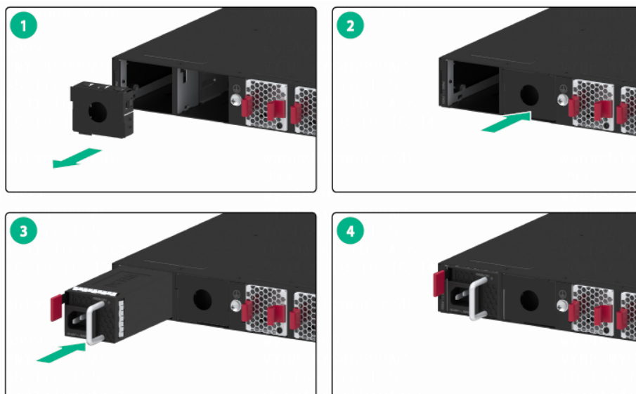
图2-9 安装电源模块
